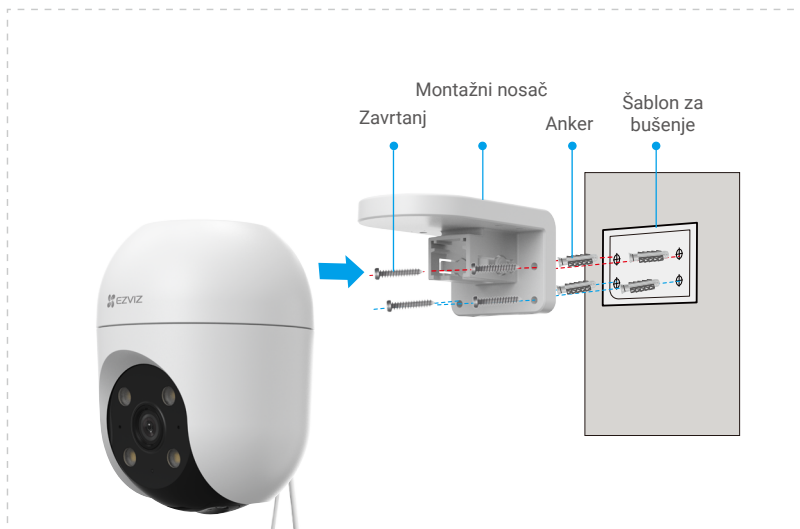
Slika 2. Montaža na zid
