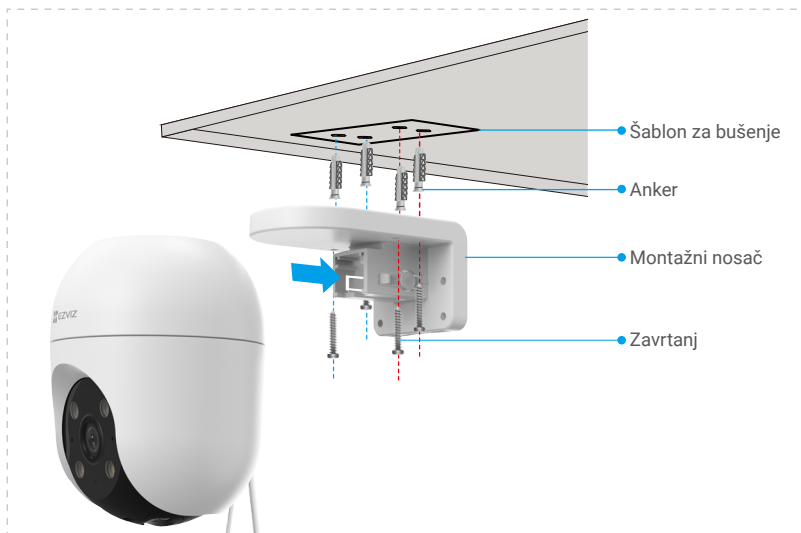
Slika 1. Montaža na plafon
